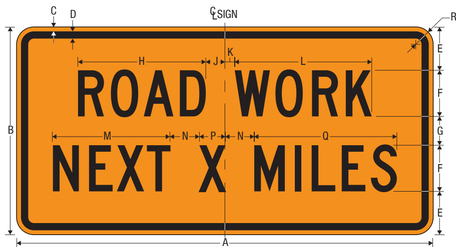
G20-1T
