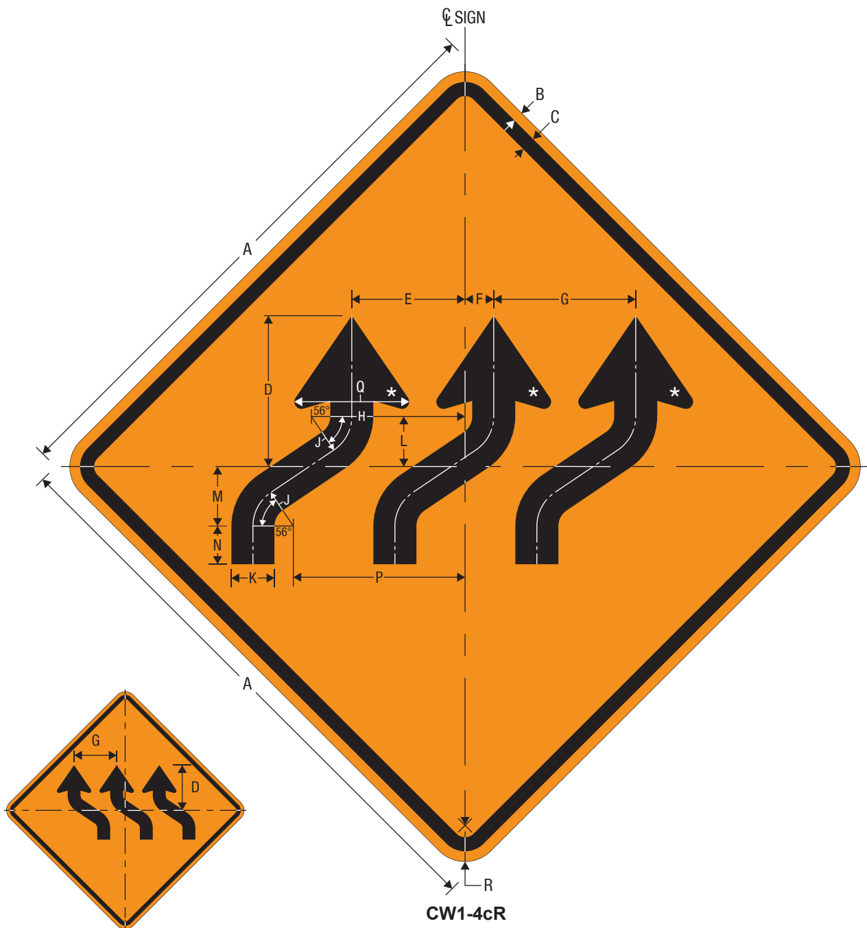
CW1-4cL
