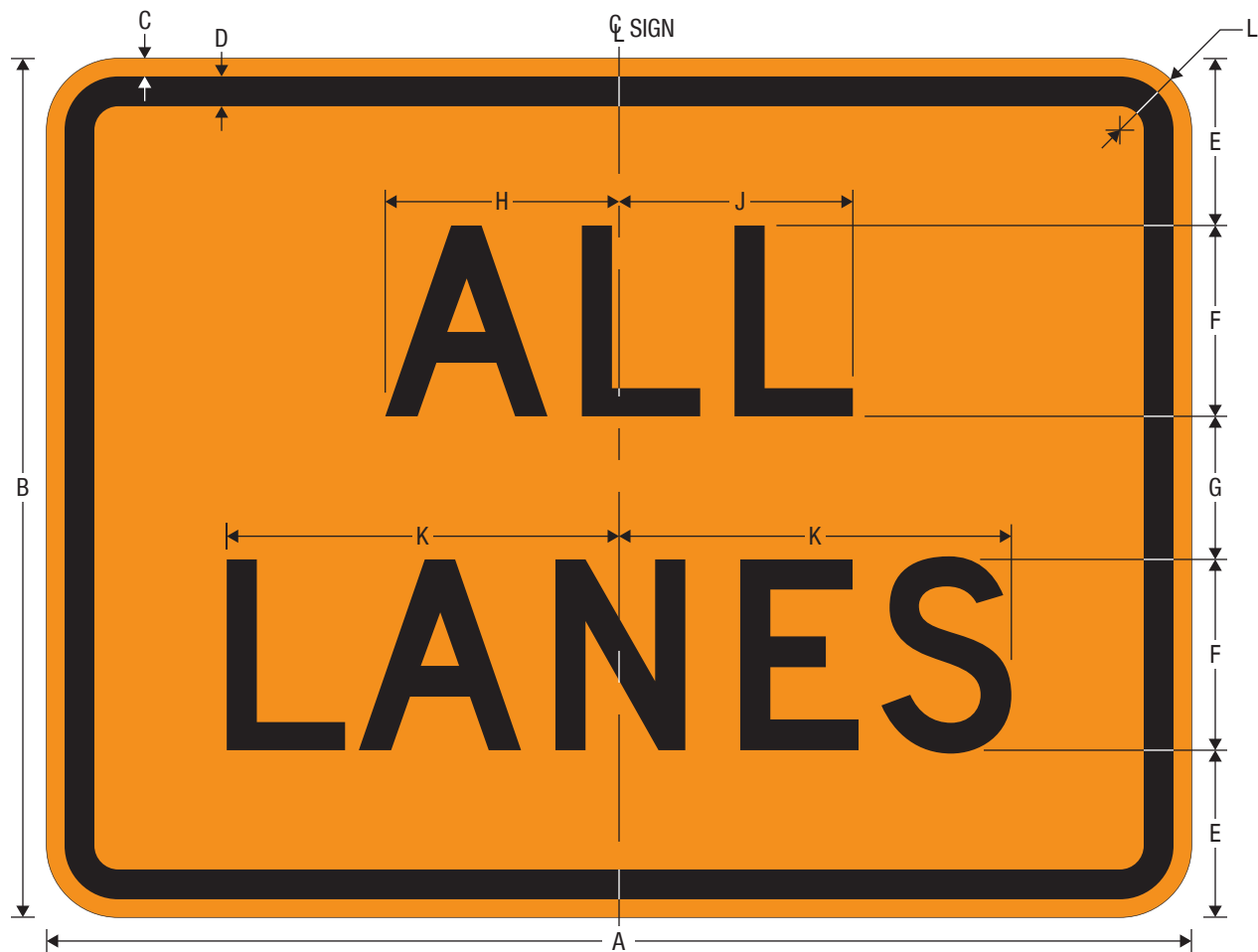
CW24-1cP ALL LANES (Plaque)
