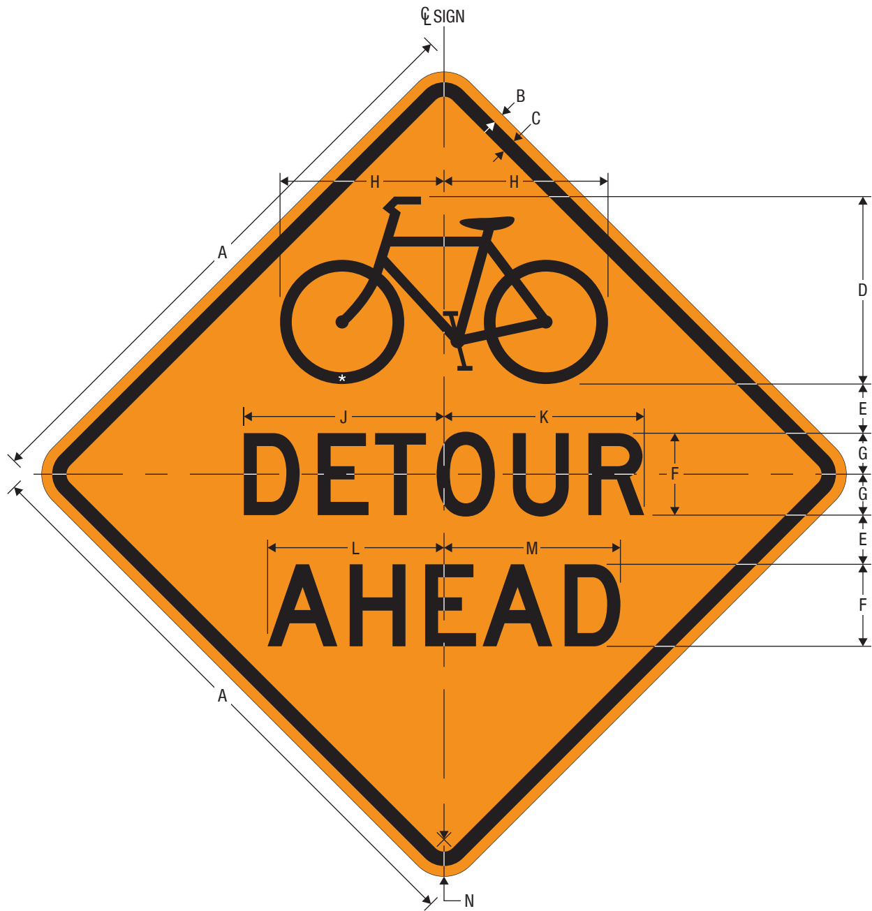
CW20-2a Bike DETOUR
