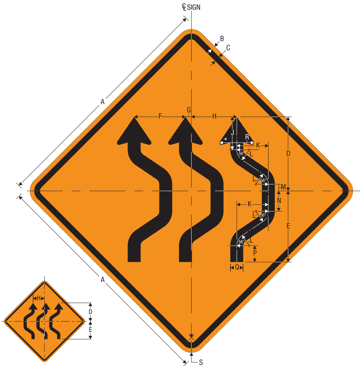
CW24-1bL
