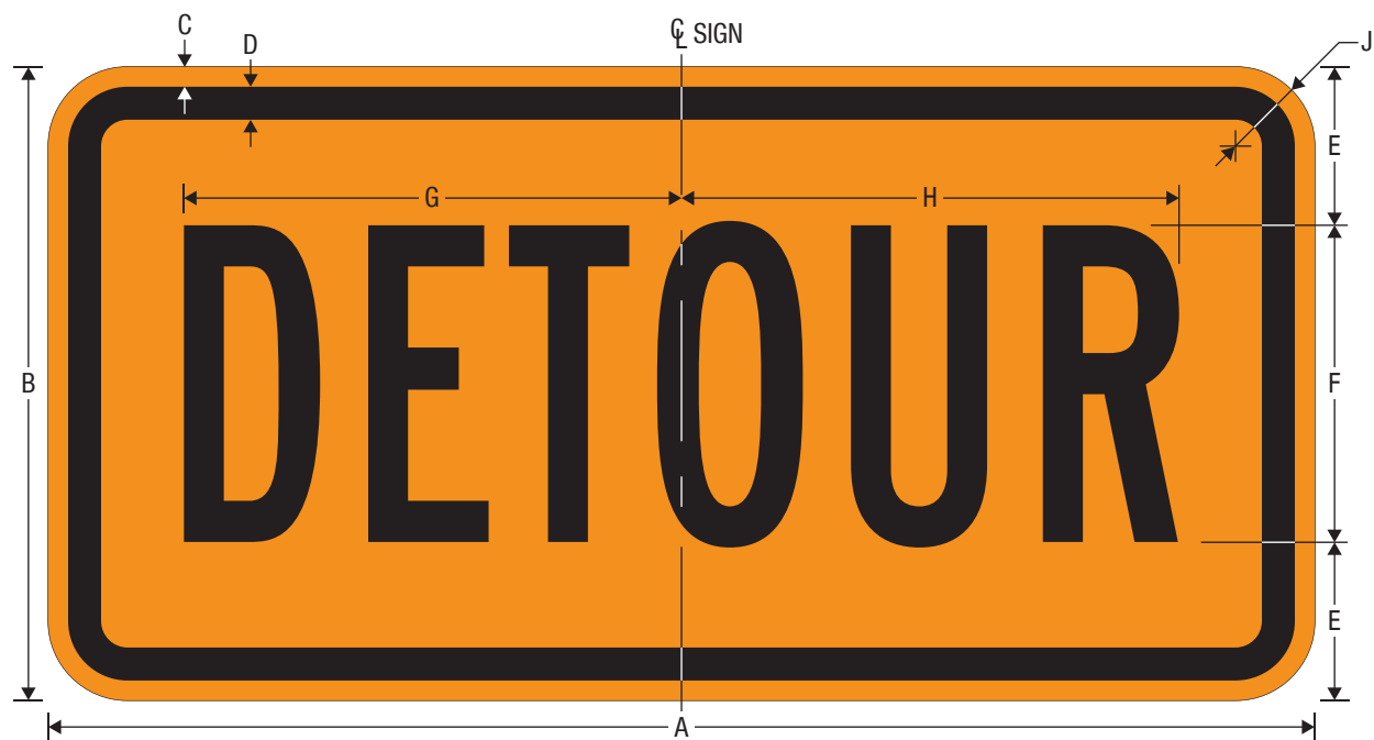
M4-8P DETOUR (Plaque)
