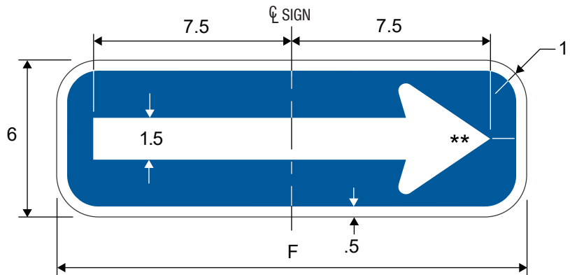
D5-5aPTR Arrow (Plaque)
