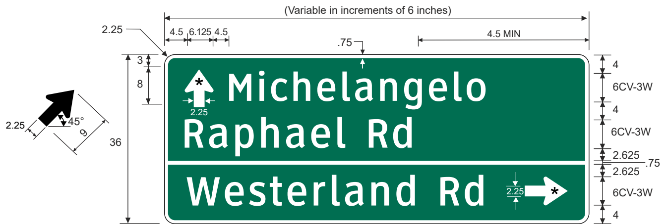
D21-3aT (UP | R)
