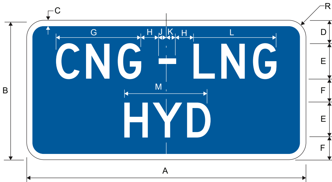
D9-11gPT CNG - LNG / HYD (Plaque)
