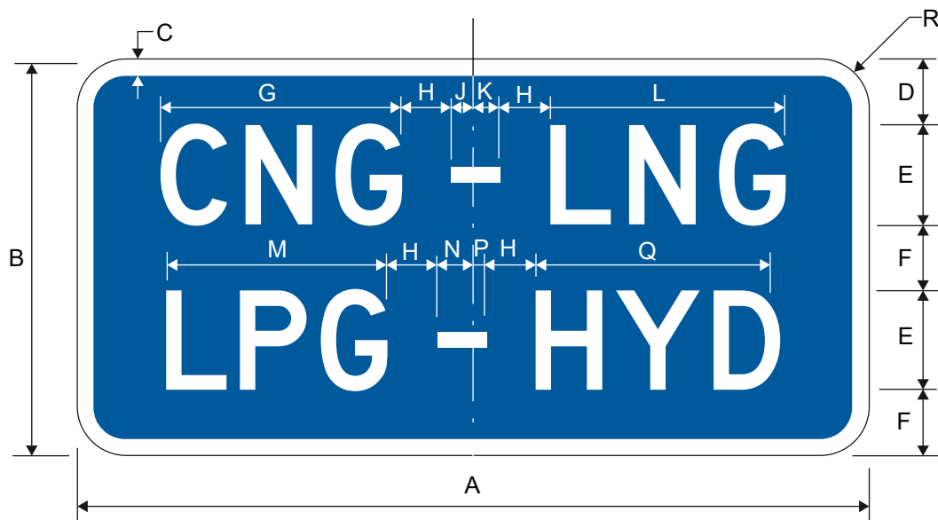
D9-11gP CNG - LNG / LPG - HYD (Plaque)
