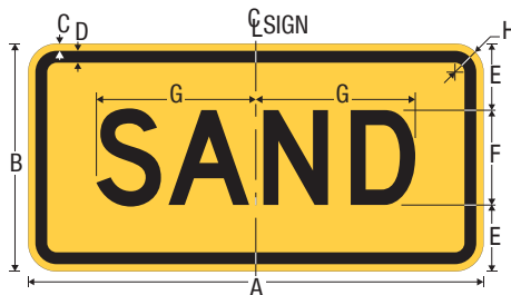
W7-4dP SAND (Plaque)
