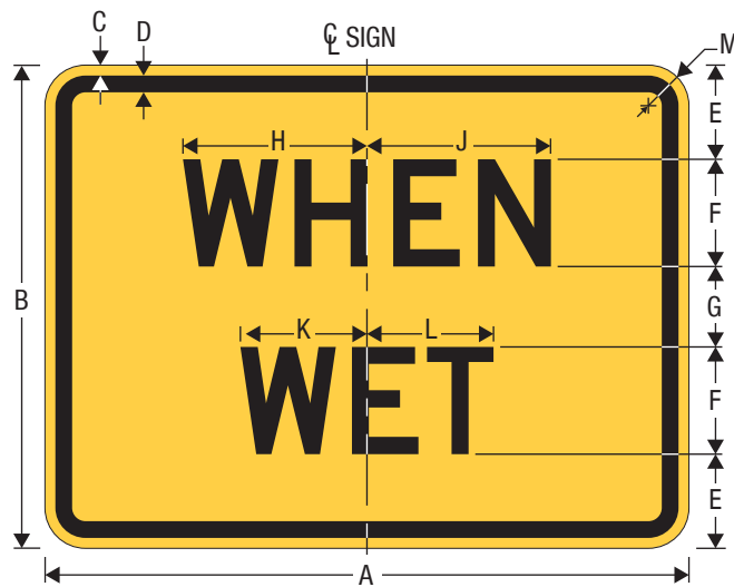
W8-5P WHEN WET (Plaque)
