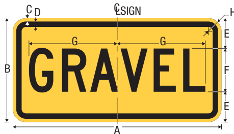
W7-4eP GRAVEL (Plaque)
