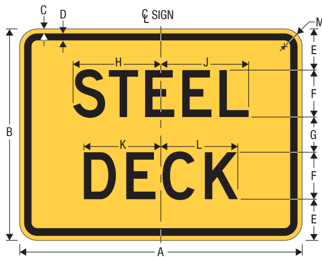
W8-5bP STEEL DECK (Plaque)
