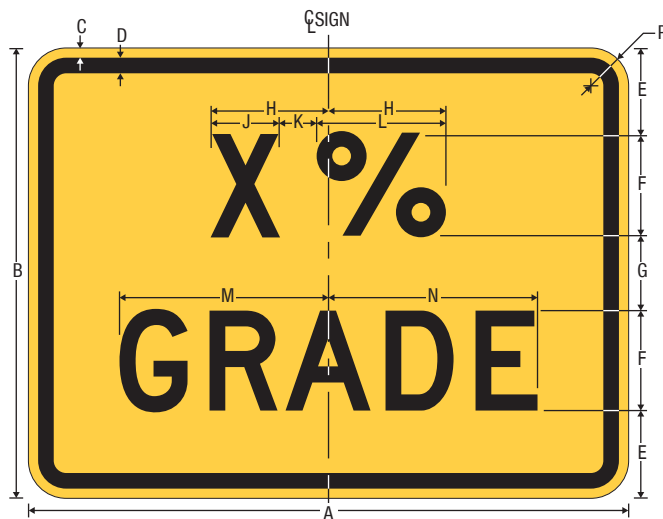
W7-3P XX% GRADE (Plaque)
