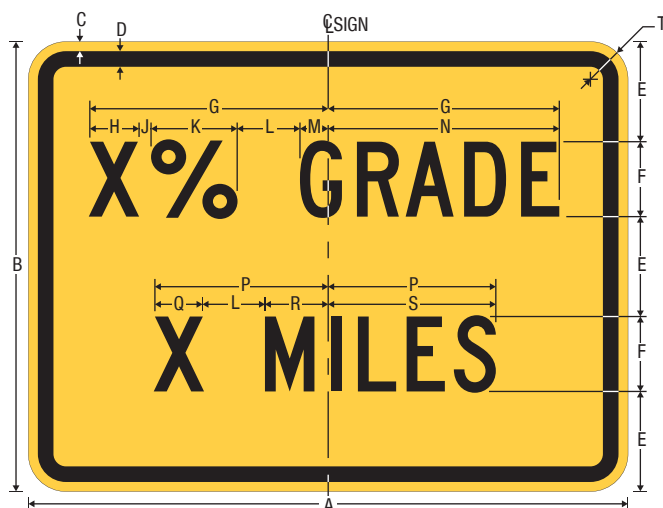
W7-3bP XX% GRADE XX MILES (Plaque)
