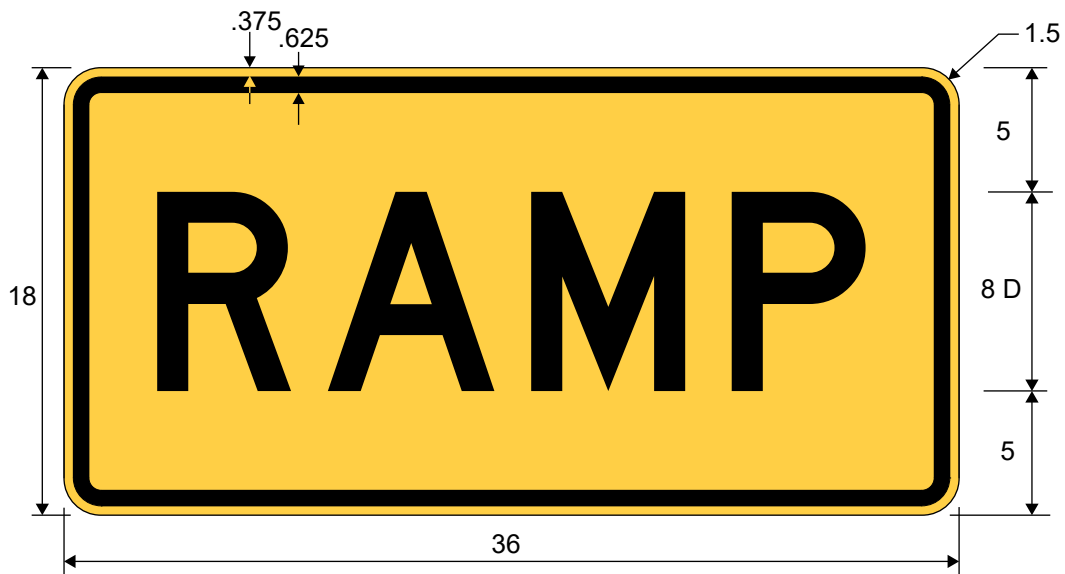
W13-4aPT RAMP (Plaque)
