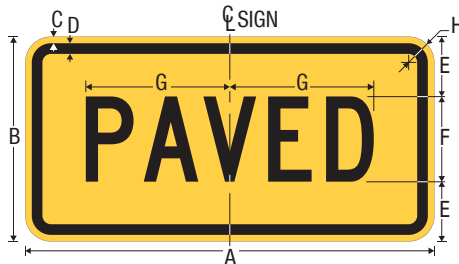
W7-4fP PAVED (Plaque)
