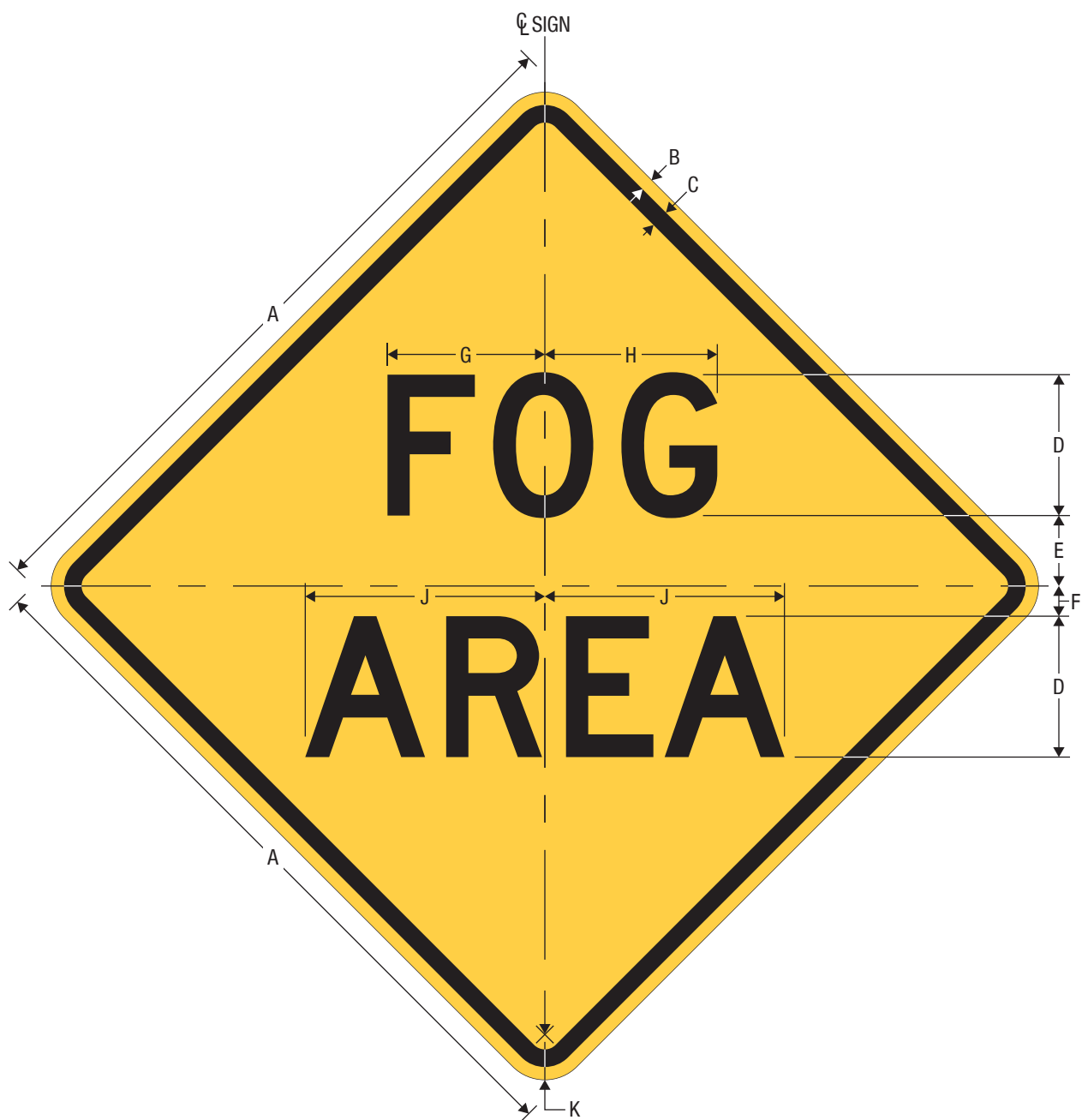
W8-22 FOG AREA
